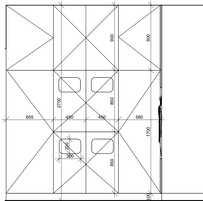
VAIZDAS IŠ PRIEKIO M1:25
