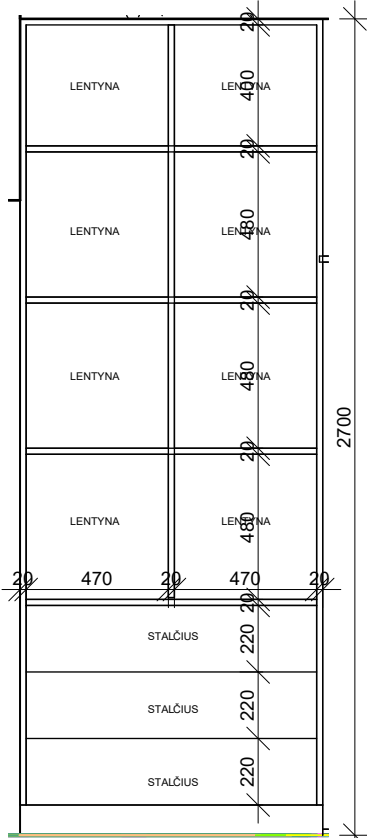
VIDAUS IŠDĖSTYMAS M 1:25
