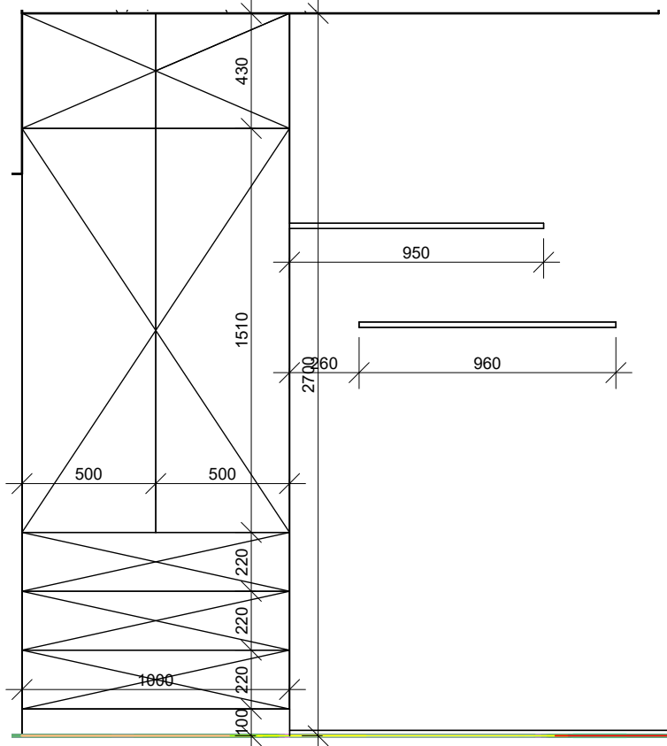
VAIZDAS IŠ PRIEKIO M 1:25
