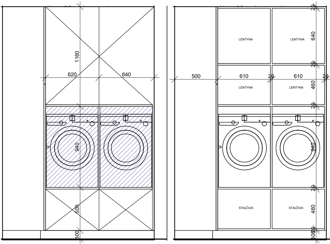
VAIZDAS IŠ PRIEKIO M1:25
